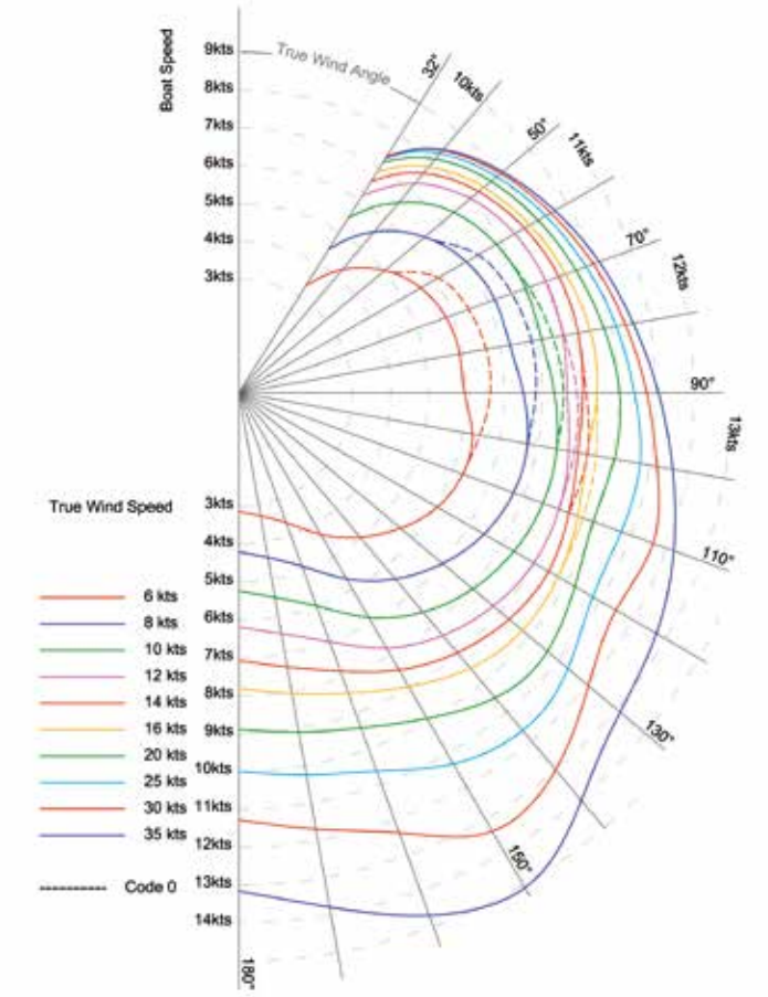
Jeanneau'nun yelken performansını polar diagram'dan inceleyebilirsiniz. Ölçüm yapılırken derin salmalı ve furling yelkenli teknede altı mürettebat var ve Code 0 da kullanıldı (üstte).
